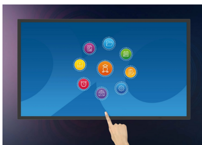
Android OS
