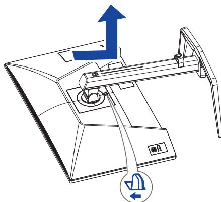
Przycisk zwalniający
