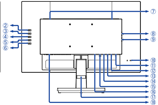
<Вид сзади>
